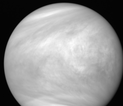
金星探査機「あかつき」が紫外線で 観測した金星 (JAXA/ISAS)
